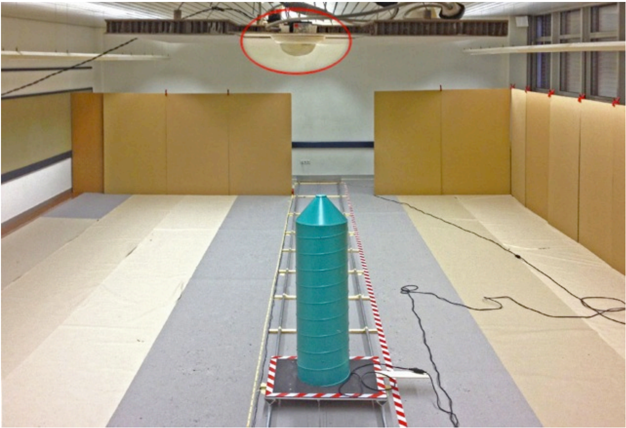
Abb. 9: Realer Messaufbau im Schulraum der HSLU
