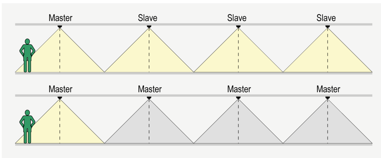
Abb. 3: Parallelschalten von PIRs erhöht die Erfassungssicherheit und mindert die Energieeinsparung
