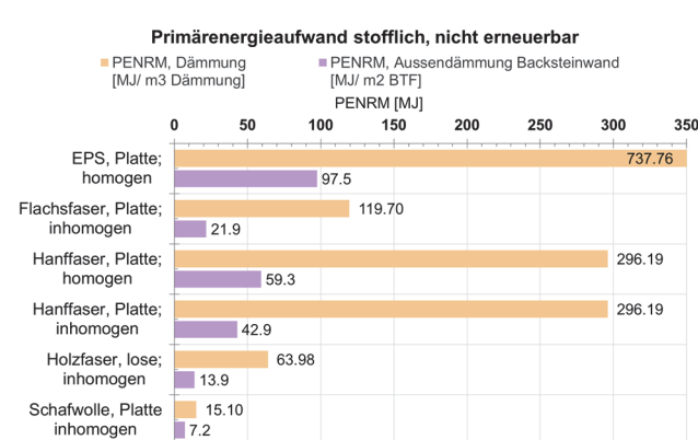
Abb.8: Materiell genutzte Primärenergie, nicht erneuerbar
