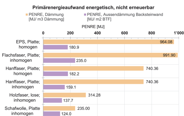
Abb.7: Energetisch genutzte Primärenergie, nicht erneuerbar
