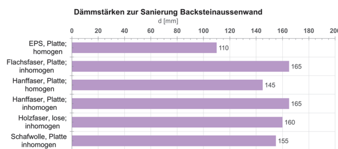
Abb. 6: Notwendige Dämmstärken
