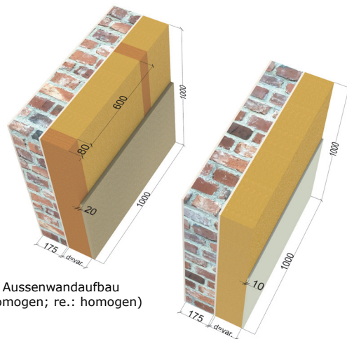
Abb. 6: Notwendige Dämmstärken
